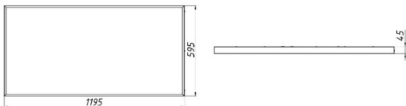
Рисунок 1а Светильник «L-office Max» встраиваемое крепление
