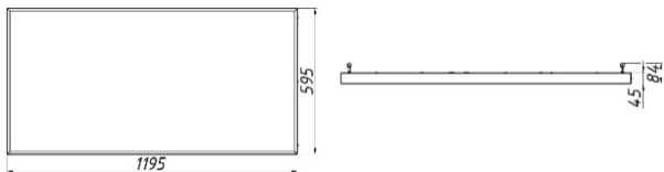
Рисунок 16 Светильник «L-office Max» подвесное крепление
